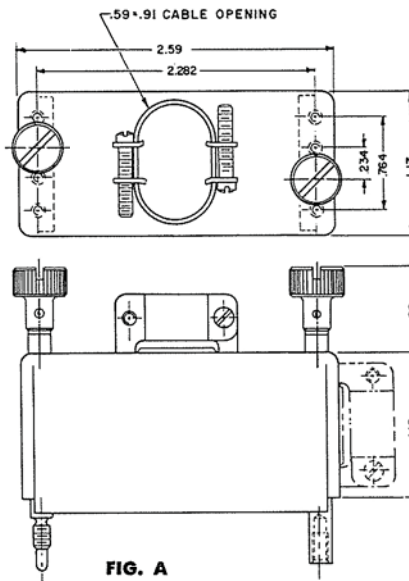
FIG. A 144 - 6 - 75 144 - 6 - 75 - 1
