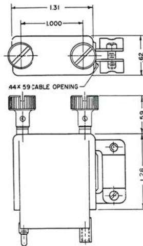
FIG. B 144 - 6 - 18 - 1
