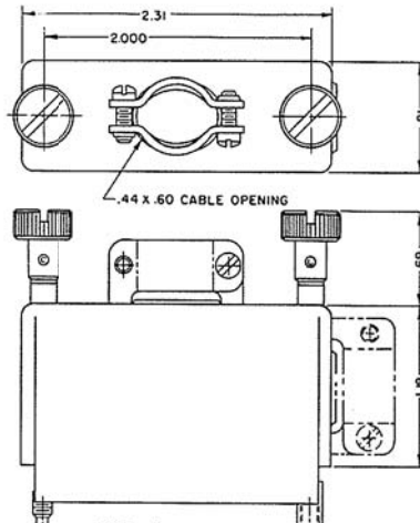
FIG. A 144 - 6 - 42 144 - 6 - 42 - 1
