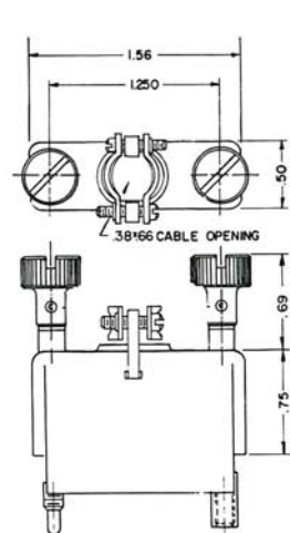
FIG. B 144 - 6 - 20
