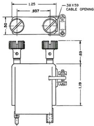
FIG. B 144 - 6 - 14 - 1
