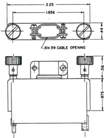
FIG. B 144 - 6 - 21
