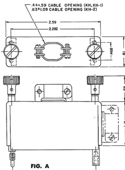
FIG. A 144 - 6 - 50 144 - 6 - 50 - 1
