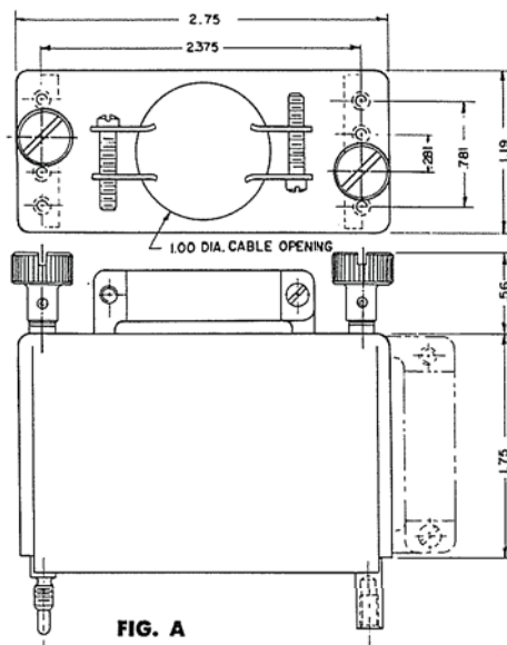
FIG. A 144 - 6 - 75 144 - 6 - 75 - 1
