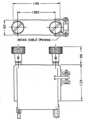
FIG. B 144 - 6 - 20 - 1
