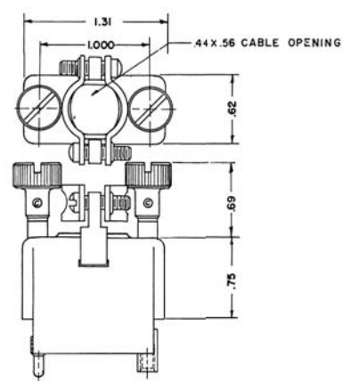
FIG. B 144 - 6 - 18
