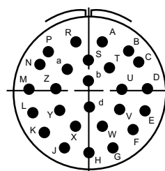
28-12 26-#16
