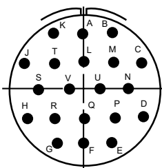
28-16 20-#16
