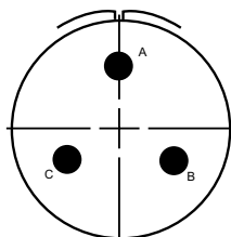
22-2 3-#8
