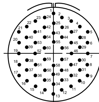
40-62 60-#16
