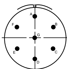
24-27 7-#16
