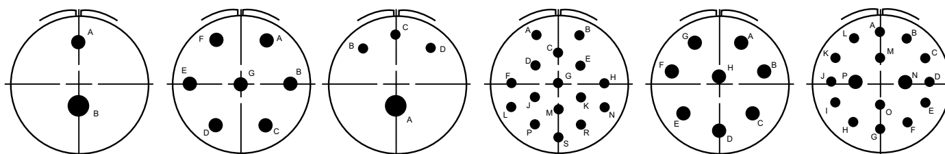
24-1 1-#12, 1-#0
