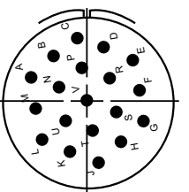
22-30 19-#16
